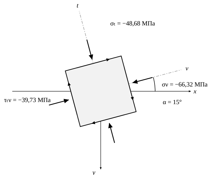
Рис. 5 — напряжения на площадках, повернутых на \alpha = 15^\circ . Оба нормальных напряжения сжимающие, стрелки направлены к граням; касательные образуют уравновешенную пару.
