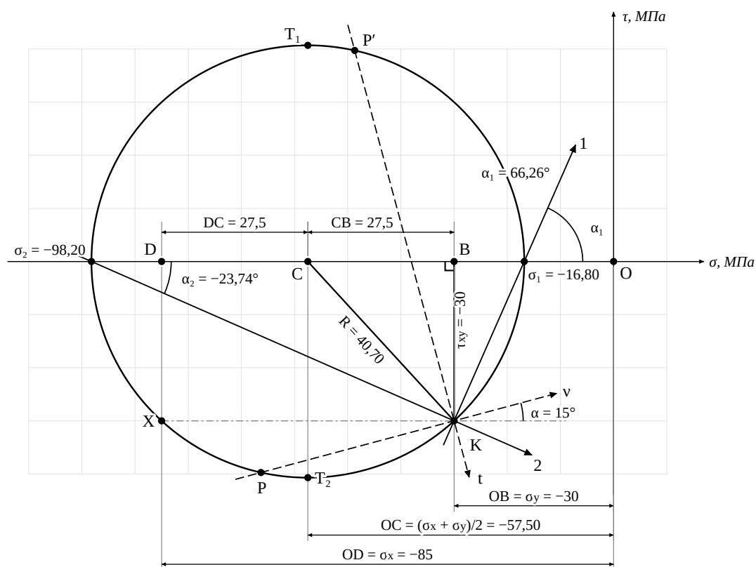
Рис. 7 — круг Мора, 1 см = 10 МПа (сетка — 10 МПа). Лучи 1 и 2 из полюса К — главные направления; T_1, T_2 — \tau_{12} = \pm 40,70 МПа при \sigma' = -57,50 МПа; Р и Р' — площадки под 15^\circ и 105^\circ : \sigma_v = -66,32 , \tau_{tv} = -39,73 ; \sigma_t = -48,68 МПа.
